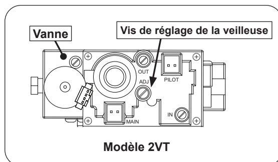
Fig. 34-4 Réglage de la veilleuse
