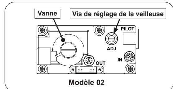
Fig. 40-3 Réglage de la veilleuse
